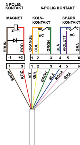
Kopplingsschema med kolv- och spärrkontakt.
